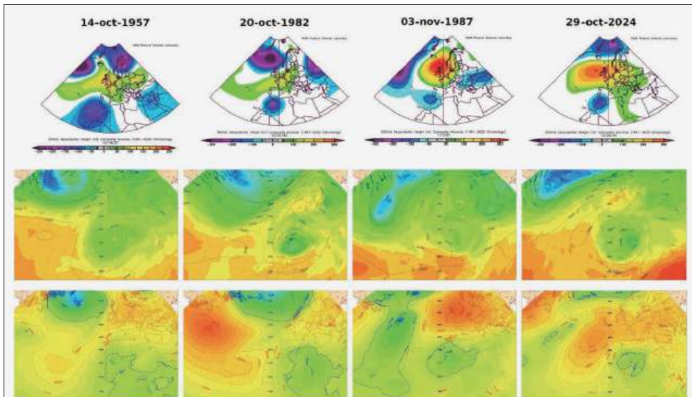
[그림 13] DANA 현상에 의한 스페인 호우 발생 시 500hPa 지위고도 편차 및 500hPa 지위고도, 해면기압 일기도
