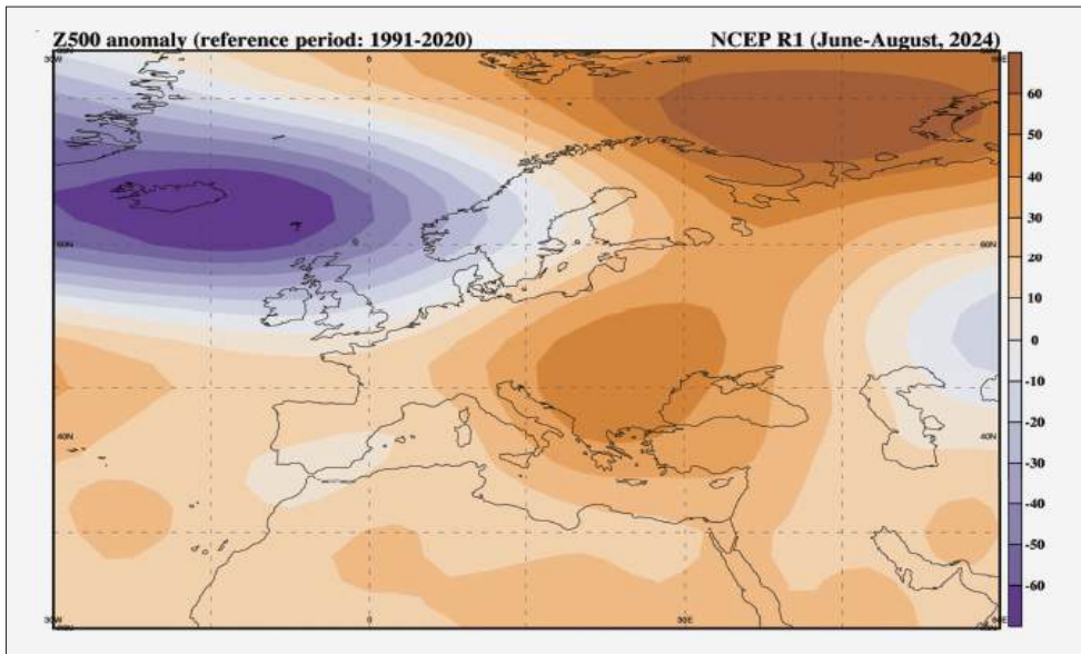
[그림 9] 2024년 6월부터 8월까지 평균한 500hPa지위고도 편차
