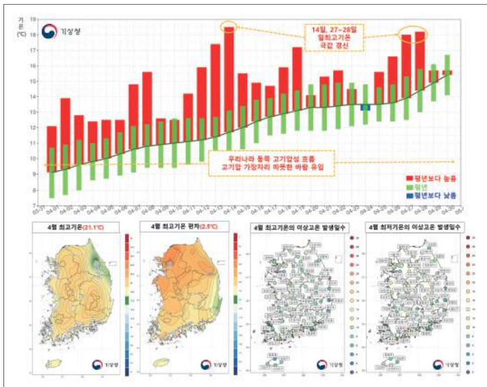
[그림 32] (위) 4월 최고기온 평년편차 일별 시계열 (아래) 4월 최고기온, 4월 최고기온 평년편차, 4월 최고기온의 이상고온 발생일수 분포도, 4월 최저기온의 이상고온 발생일수 분포도
