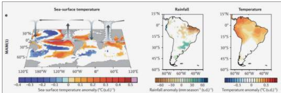
[그림 25] 엘니뇨 발생 이후 3~5월 평균(MAM)전지구 해수면온도, 워커 순환과 남미의 강수, 기온 반응 ※ 출처: Cai et al. 2020
