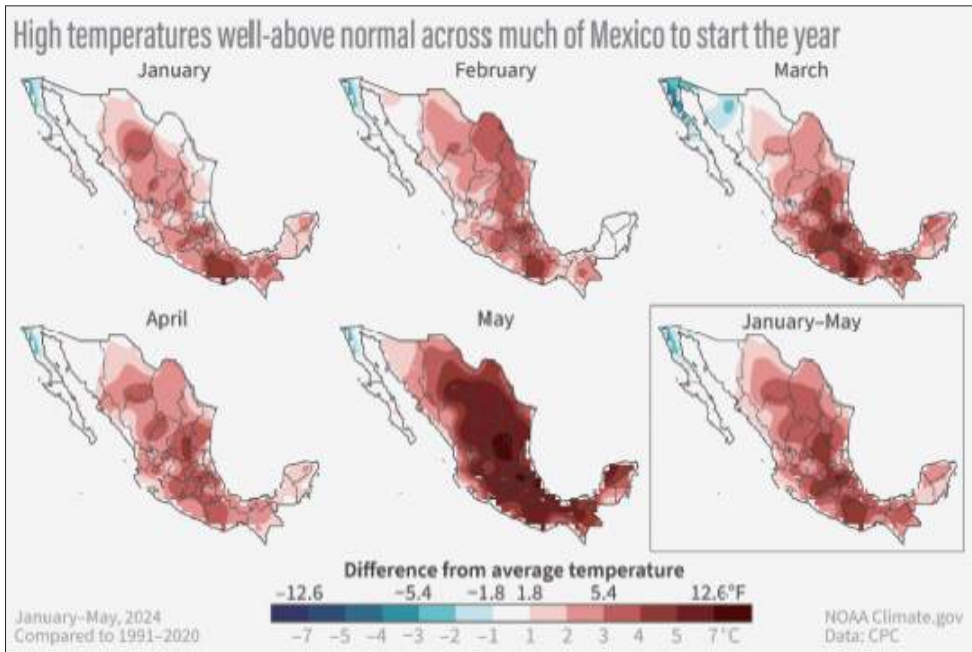
[그림 28] 1~5월 멕시코 기온 편차 ※ 출처: NOAA Climate.gov
